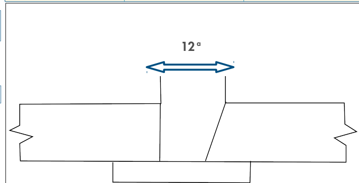
Figuur 1: Gecombineerd proefstuk voor hoeklas en stompe las. Hierbij valt op dat er gebruik gemaakt wordt van een backingstrip, waardoor de kwalificatie voor de stompe naad enkel met backing is
